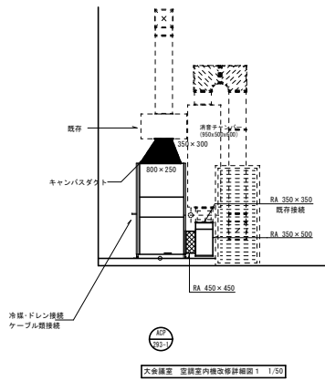
大会議室 空調室内機改修詳細図 1 1/50
