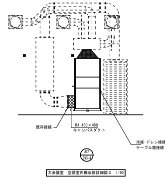
大会議室 空調室内機改修詳細図 2 1/50
