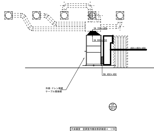
大会議室 空調室内機改修詳細図 4 1/50
