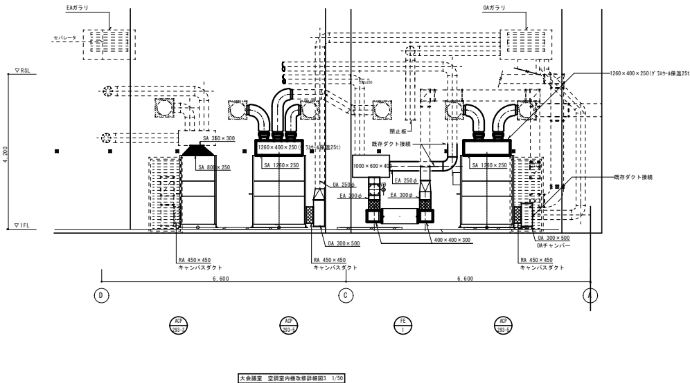
大会議室 空調室内機改修詳細図 3 1/50
